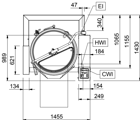
Boven aanzicht
